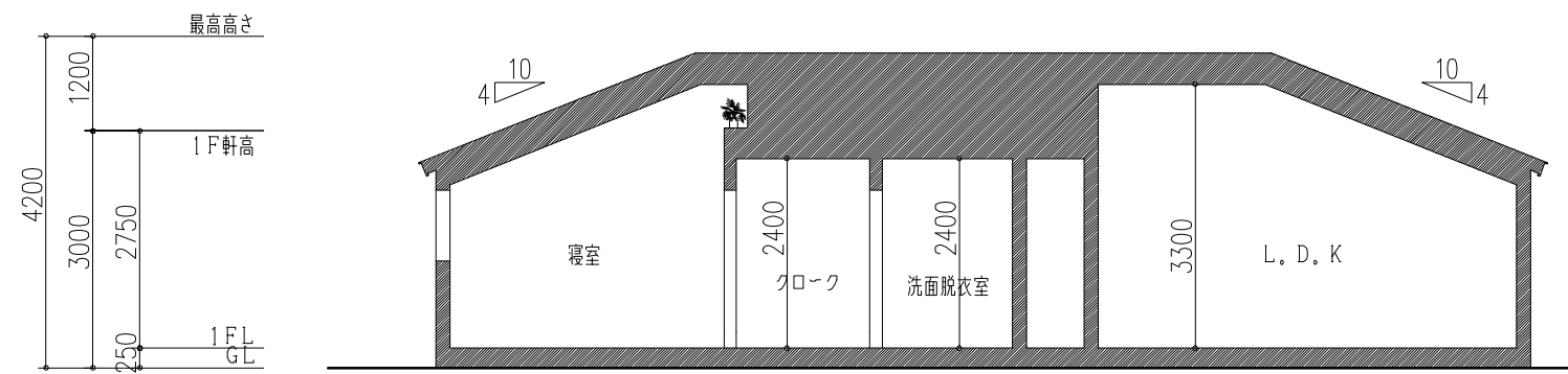
A-A' 断面図 1:100
