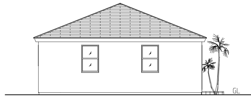
東立面図 1:100
