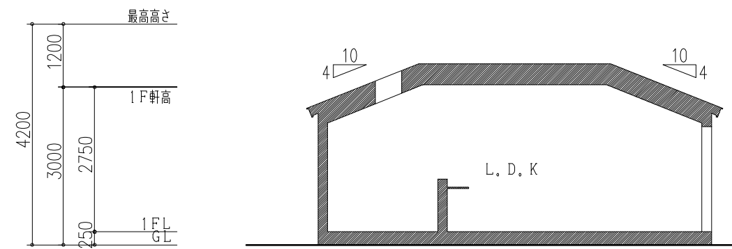
B-B' 断面図 1:100
