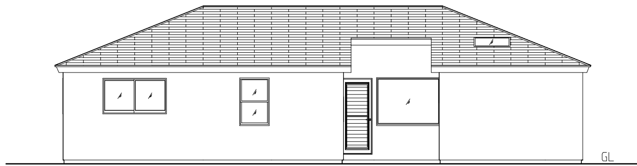
南立面図 1:100
