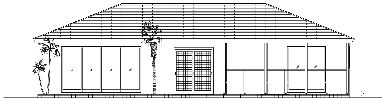
北立面図 1:100
